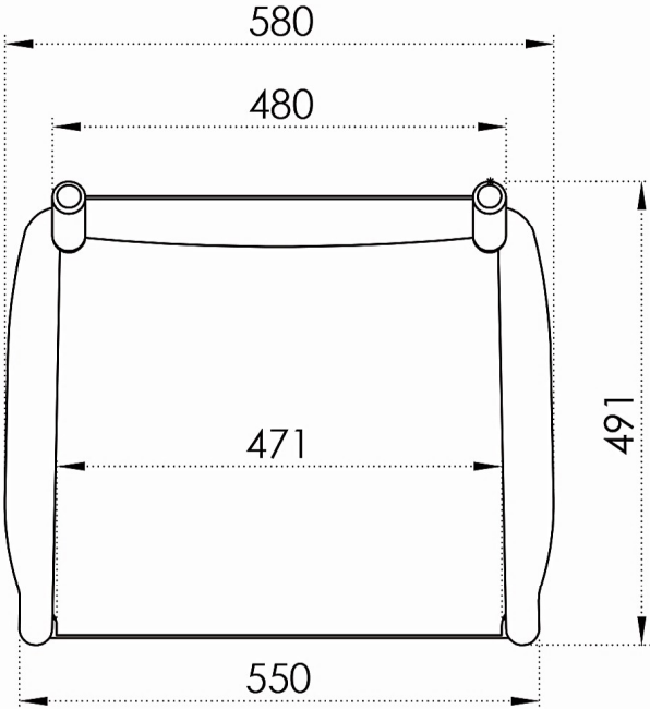
VISTA SUPERIOR
