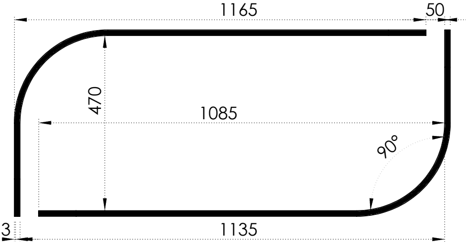
VISTA SUPERIOR
