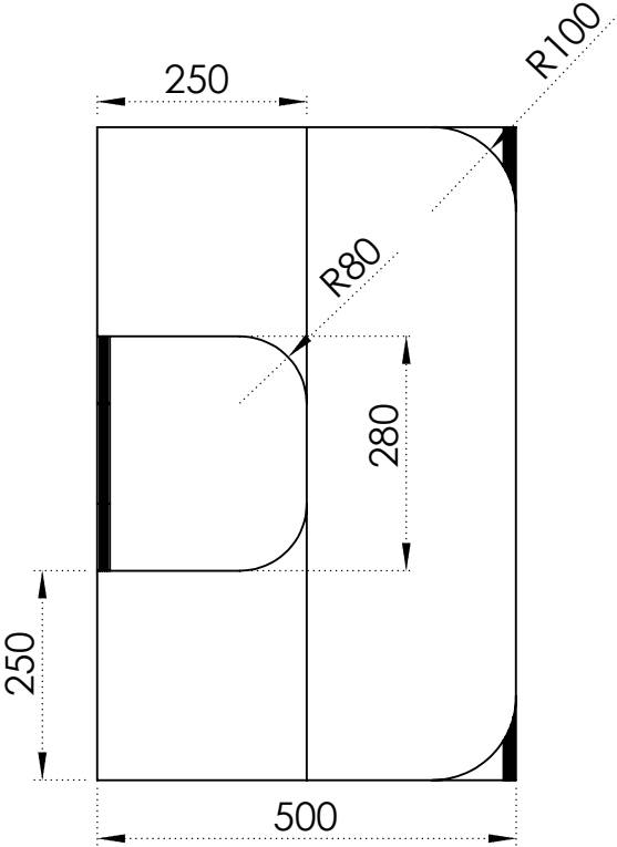
VISTA LATERAL
